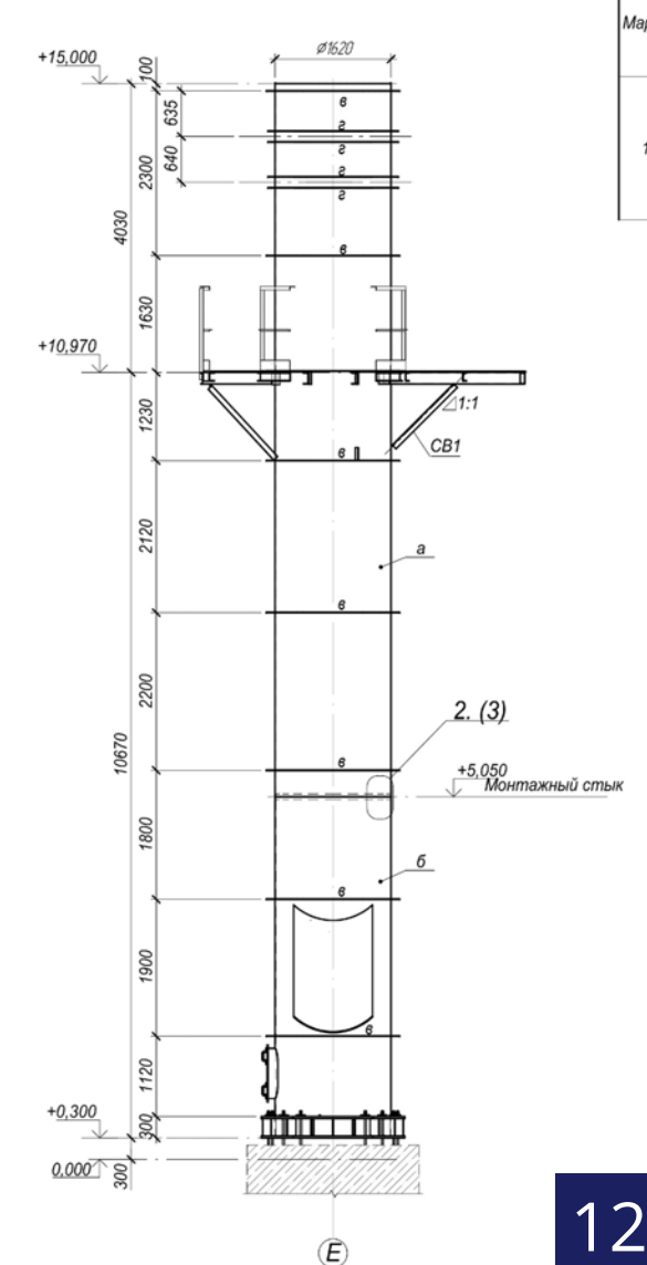
Разрез 2 - 2
